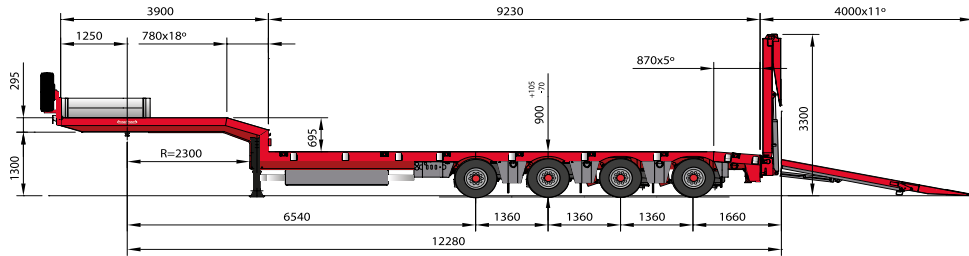
OSD-73-04V(S)
