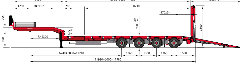
OSD-73-04V(SN2520)
