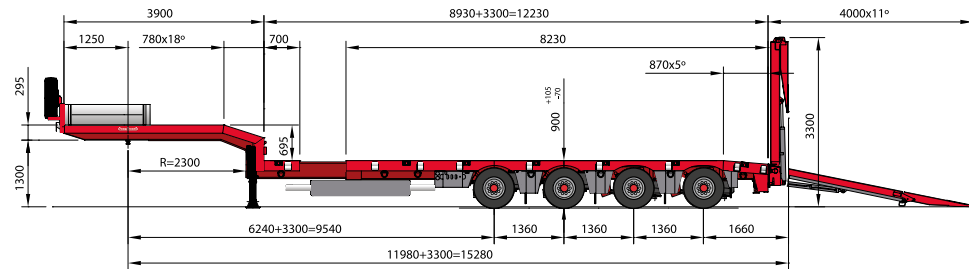
OSD-73-04V(SN)
