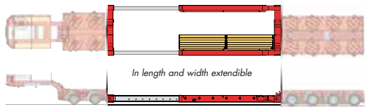
Cama portatubos, deslizable en anchura con piso de madera desmontable
