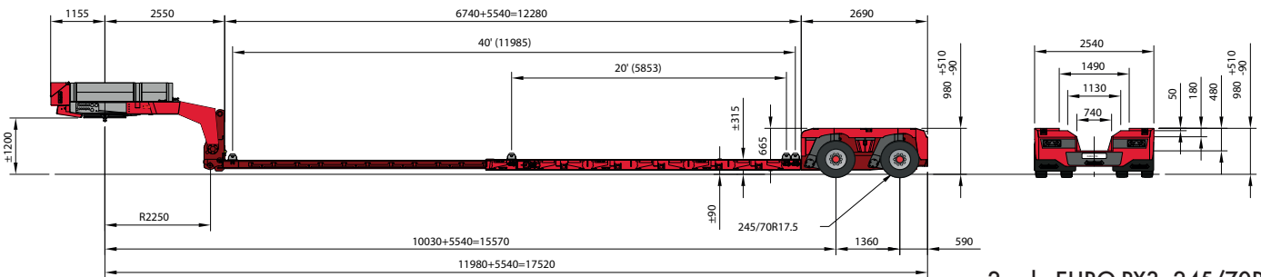
2-axle EURO-PX3: 245/70R17.5 tires
