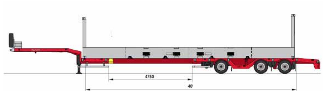
GELADEN MET EEN 40-VOET FLATRACK
