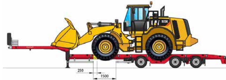
GELADEN MET EEN CATERPILLAR 972K WIELLADER
