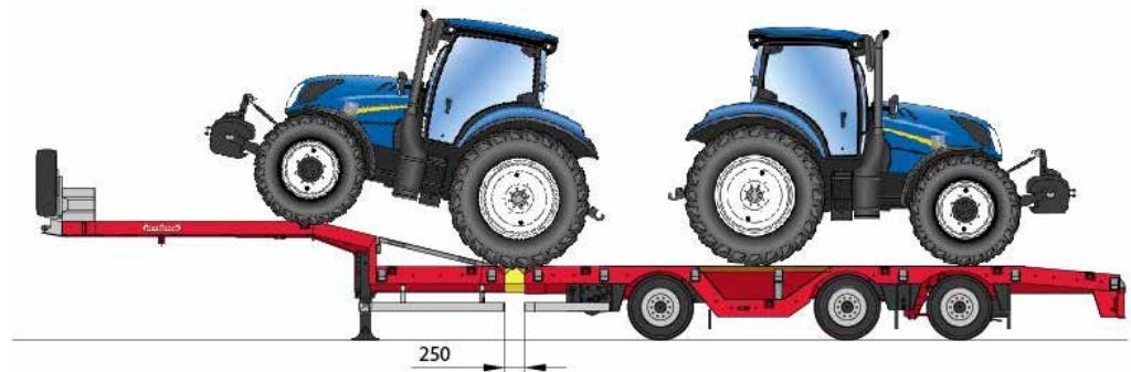
GELADEN MET TWEE NEW HOLLAND T6 AGRARISCHE TRACTOREN
