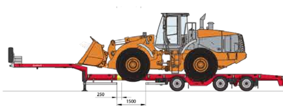
GELADEN MET EEN HITACHI ZW310 WIELLADER
