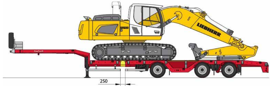
GELADEN MET EEN LIEBHERR R-926 RUPSGRAAFMACHINE
