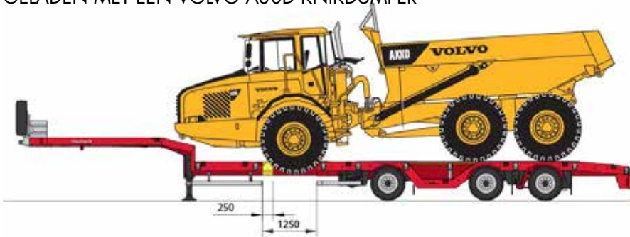
GELADEN MET EEN VOLVO A30D KNIKDUMPER
