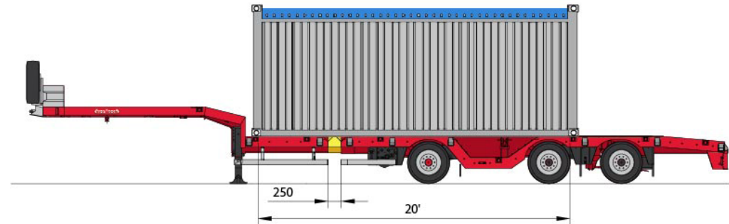
GELADEN MET EEN ISO 20-VOET CONTAINER
